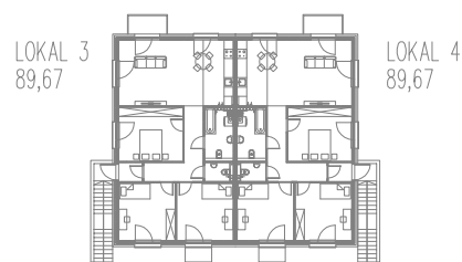
PIĘTRO
